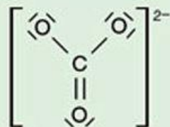
\text{CO}_3^{2-} , ione carbonato
