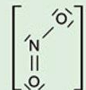
\text{NO}_2^- , ione nitrito
