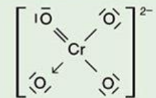
CrO 4 2- , ione cromato
