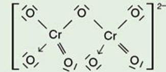
Cr 2 O 7 2- , ione dicromato
