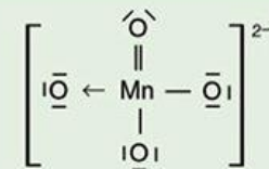
MnO 4 2- , ione manganato
