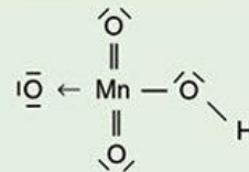
HMnO 4 , acido permanganico
