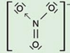
NO 3 - , ione nitrato
