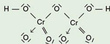
H 2 Cr 2 O 7 , acido dicromico
