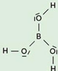
\text{H}_3\text{BO}_3 , acido (orto)borico
