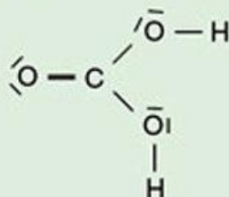
\text{H}_2\text{CO}_3 , acido carbonico**
