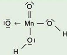
H 2 MnO 4 , acido manganico
