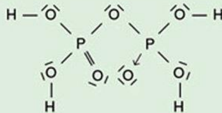
H 4 P 2 O 7 , acido pirofosforico
