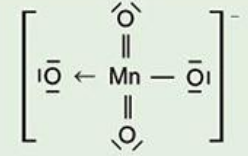
MnO 4 - , ione permanganato
