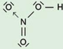
HNO 3 , acido nitrico
