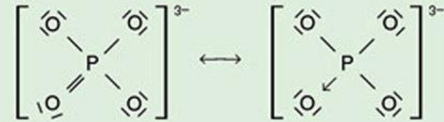
PO 4 3- , ione (orto)fosfato
