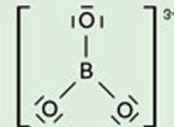
\text{BO}_3^{3-} , ione borato
