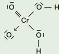
H 2 CrO 4 , acido cromico
