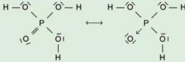
H 3 PO 4 , acido (orto)fosforico
